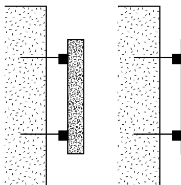
← Rys. 14. Przekrój poprzeczny mocowania szyny z szyldem.
