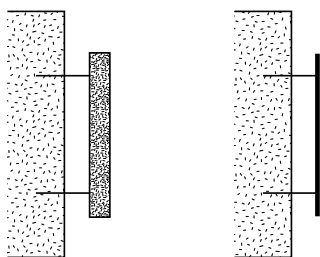
↑ Rys. 17. Przekrój poprzeczny mocowania na szpilkach.
