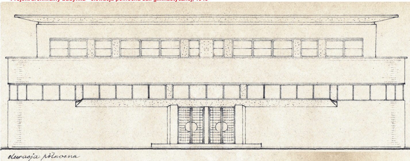
Projekt archiwalny budynku - elewacja północna sali gimnastycznej, 1948
