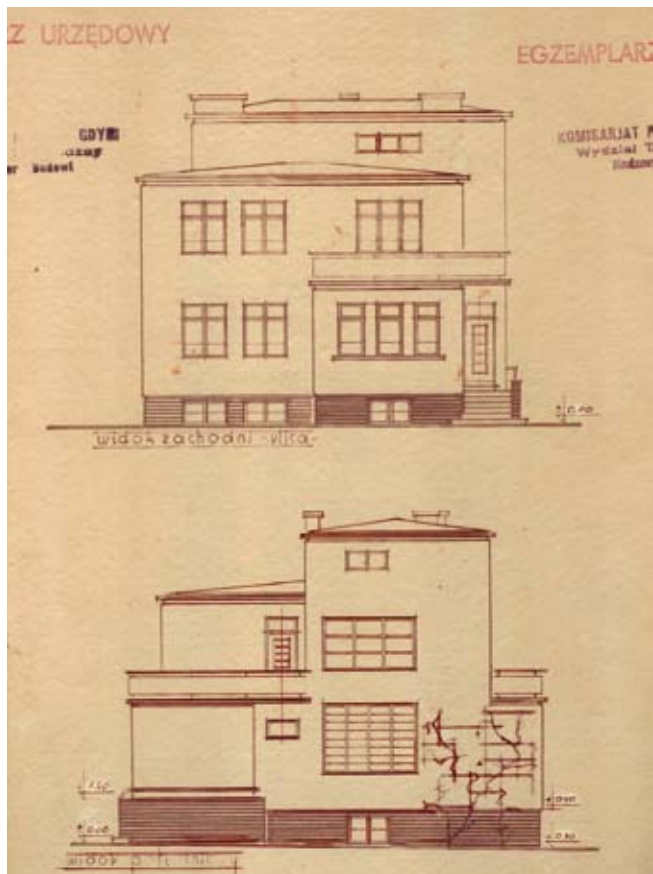
Willa w Orłowie Gdynia, ul. Inżynierska 111 projektant: Narcyz Obrycki, 1936 r.
