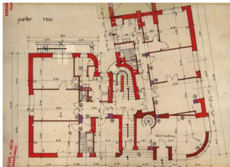
Budynek mieszkalny, Gdynia, ul. Słupecka 9 projektant: Stanisław Ziółowski, 1937 r.
